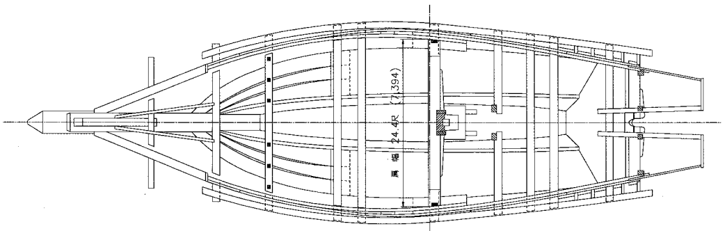
平面図 (下回り)
