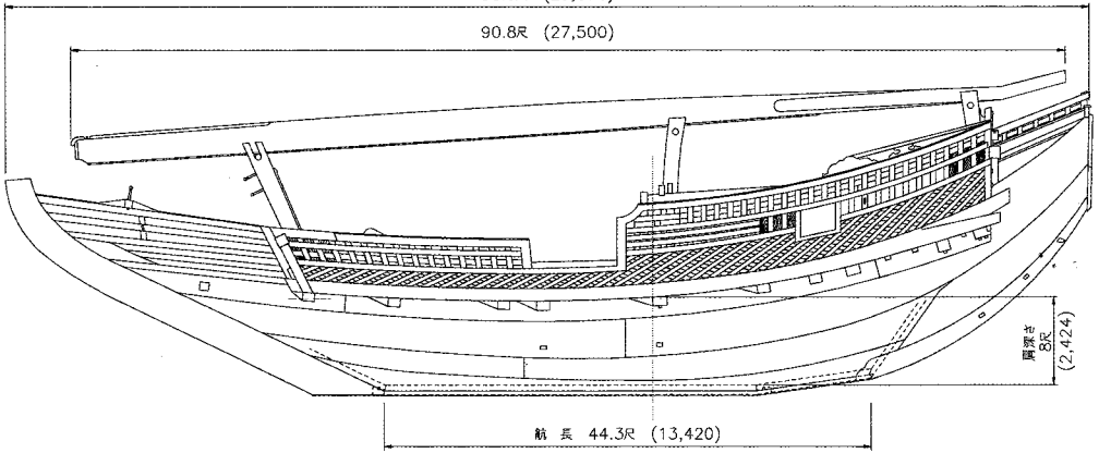
側面図
