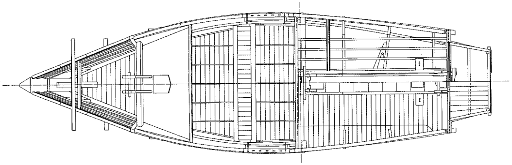
平面図 (上回り)
